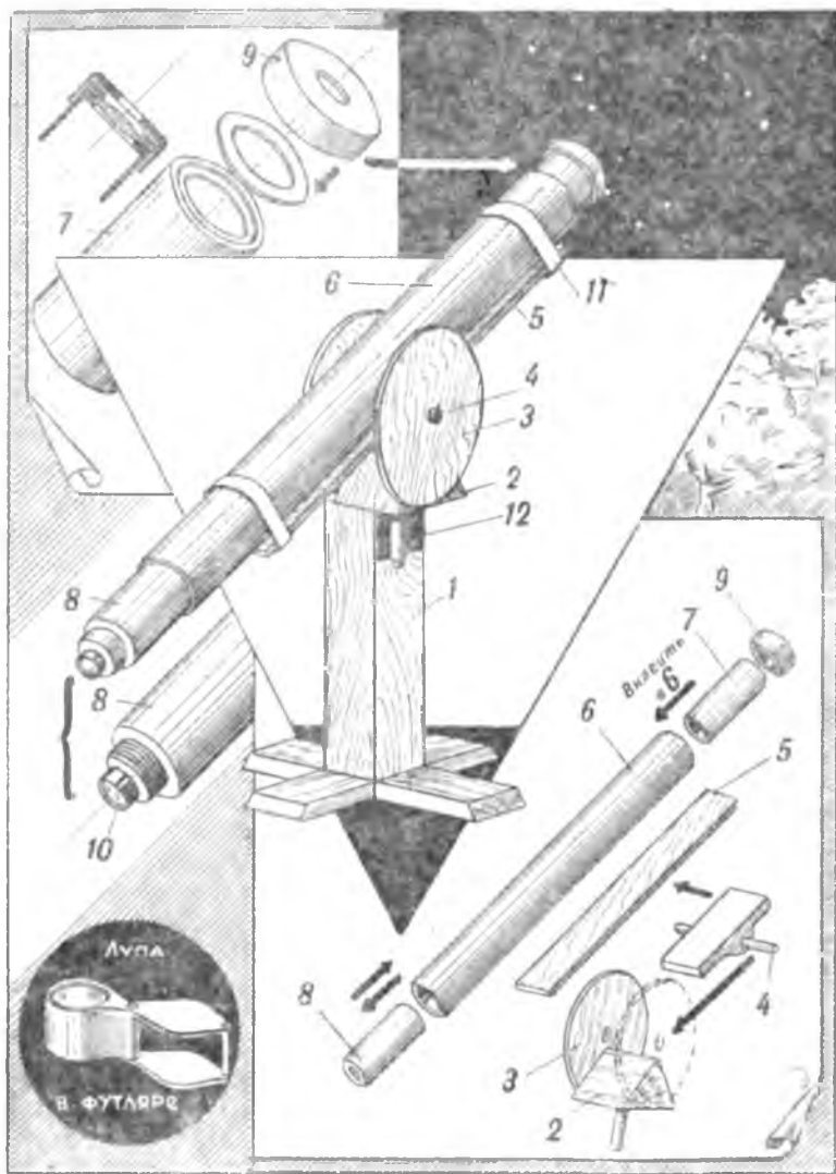
Т а б л и ц а 4 Телескоп. 1 — стойка; 2 — треугольник; 3 — фанерный кружок; 4 — поперечная ось; 5 — линейка; 6 — труба; 7 — коробка с объективом; 8 — коробка с окуляром; 9 — крышка с диафрагмой объектива; 10 — трубка окуляра; 11 — матерчатая лента; 12 — обойма вертикальной оси.
