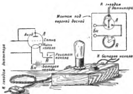
Т а б л и ц а 13. Ламповый детектор.
