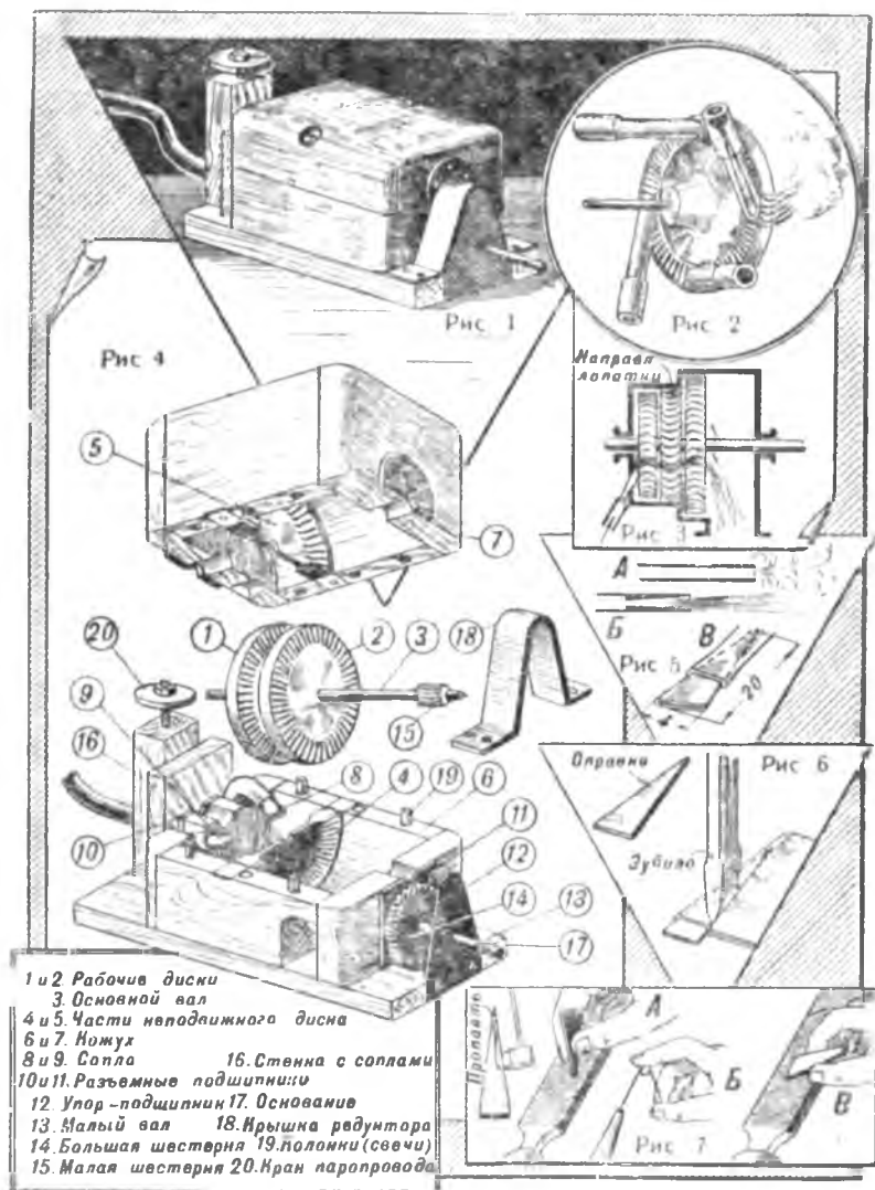
Т а б л и ц а 36. Конструкция паровой турбины.
