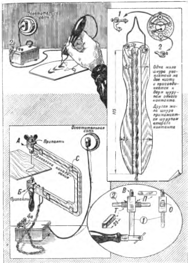
Т а б л и ц а 29. Электровыжигатель и электролобзик.
