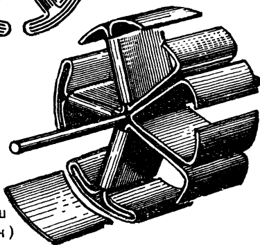
Рис. 39. Щеткодержатель со щетками и сердечник якоря.
