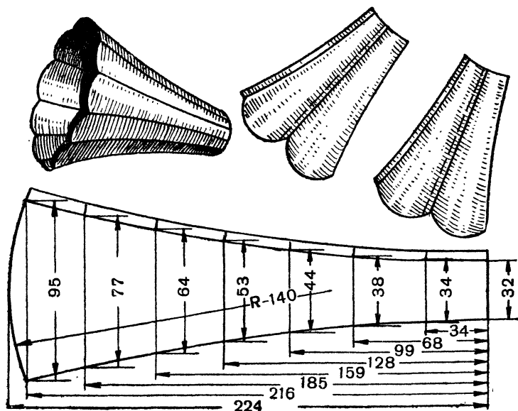
Рис. 27. Рупор.
