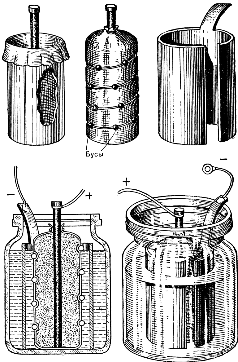
Рис. 30. Гальванические элементы.
