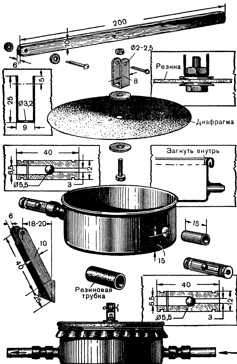
Рис. 10. Детали насоса-«лягушки».
