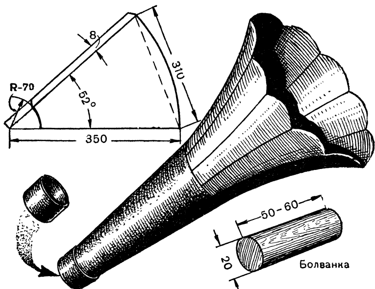
Рис. 28. Горловина рупора.
