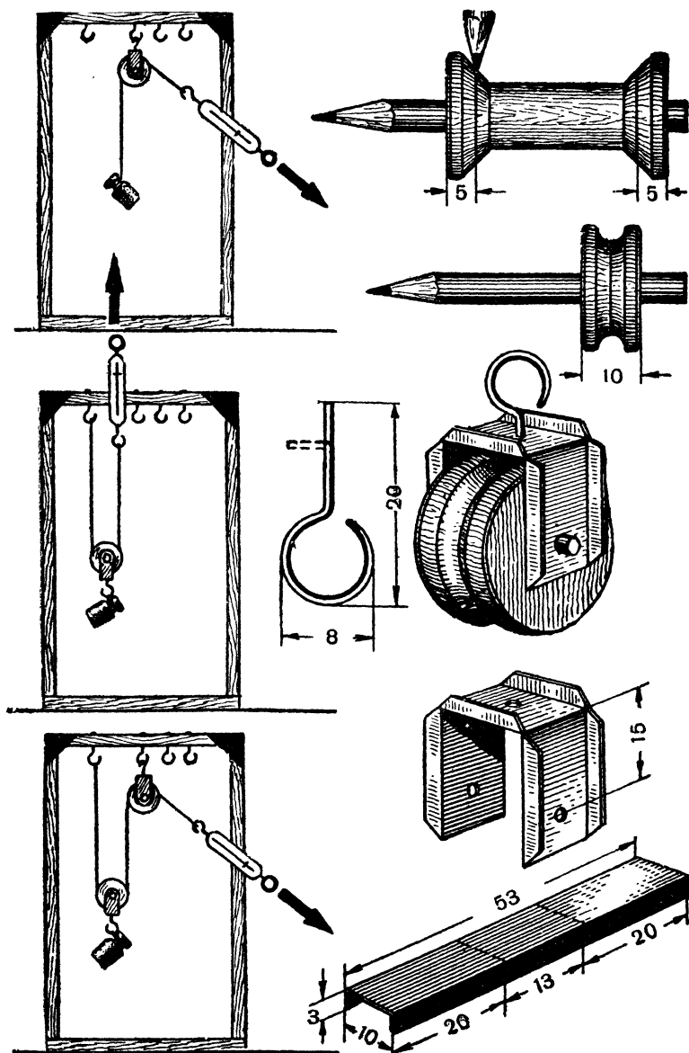
Рис. 19. Блоки.
