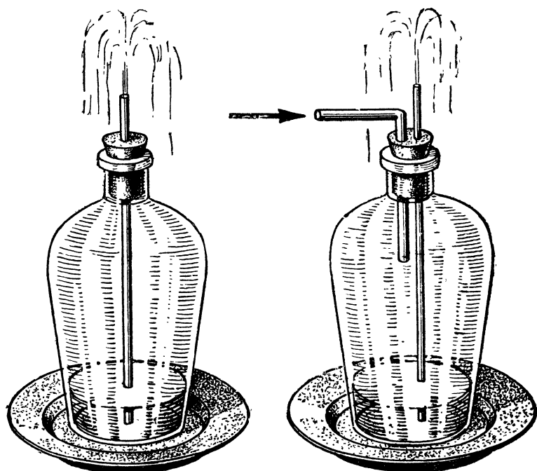
Рис. 7. Геронов фонтан.
