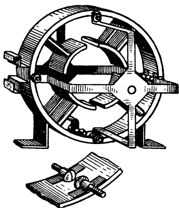
Рис. 37. Крепление крестовин к статору.
