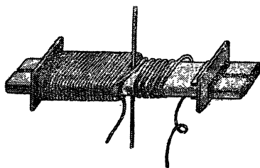
Рис. 22. Обмотка якоря.
