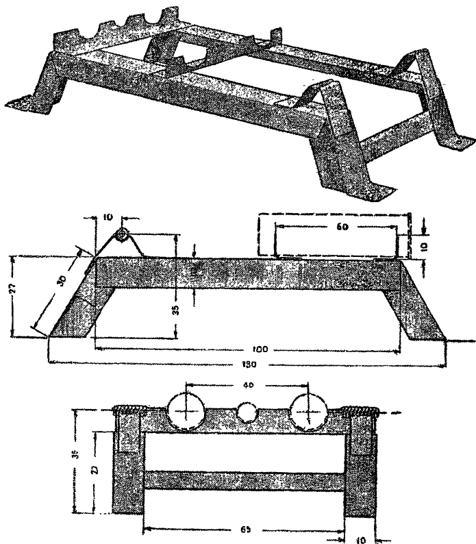
Рис. 108. Изготовление фермы.
