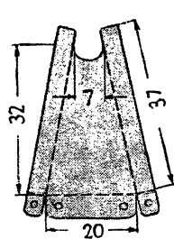
Рис. 87. Развертки опор.
