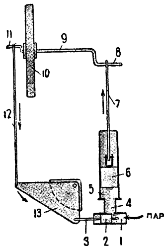
Рис. 84. Наверху — схема работы одноцилиндровой машины (вид сбоку), внизу — вид машины сверху: 1 — трубка золотника, 2 — поршень золотника, 3 — шток золотника, 4 — соединительная трубочка, 5 — цилиндр машины, 6 — поршень, 7 — шатун поршня, 8 — кривошип вала, 9 — вал, 10 — маховое колесо, 11 — второй кривошип, 12 — тяга треугольника, 13 — треугольник.
