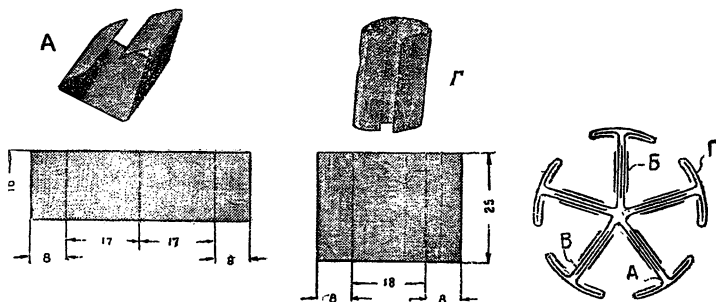
Рис. 65. Основные детали и конструкция пятиполюсного якоря.
