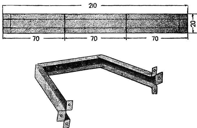
Рис. 31. Изготовление профилированной стойки.
