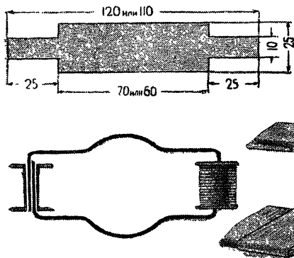
Рис. 47. Конструкция статора.
