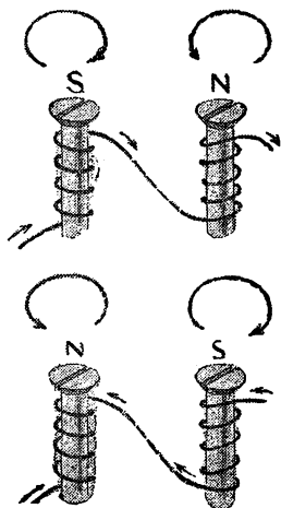
Рис. 19. Полюсы электромагнита перемагничиваются при изменении направления тока.
