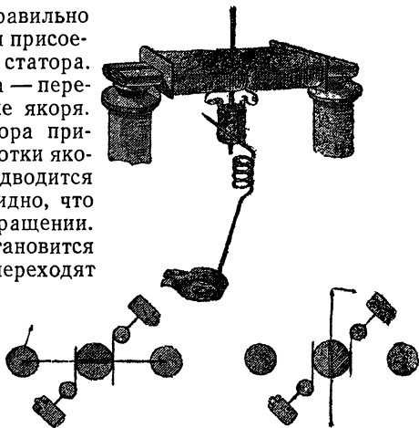
Рис. 25. При вращении якоря коллектор переключает ток.
