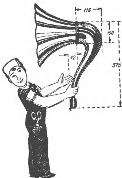
Рис. 21. Размеры изогнутого рупора.
