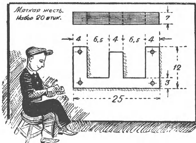
Рис. 45. Сердечник «Рекорда».
