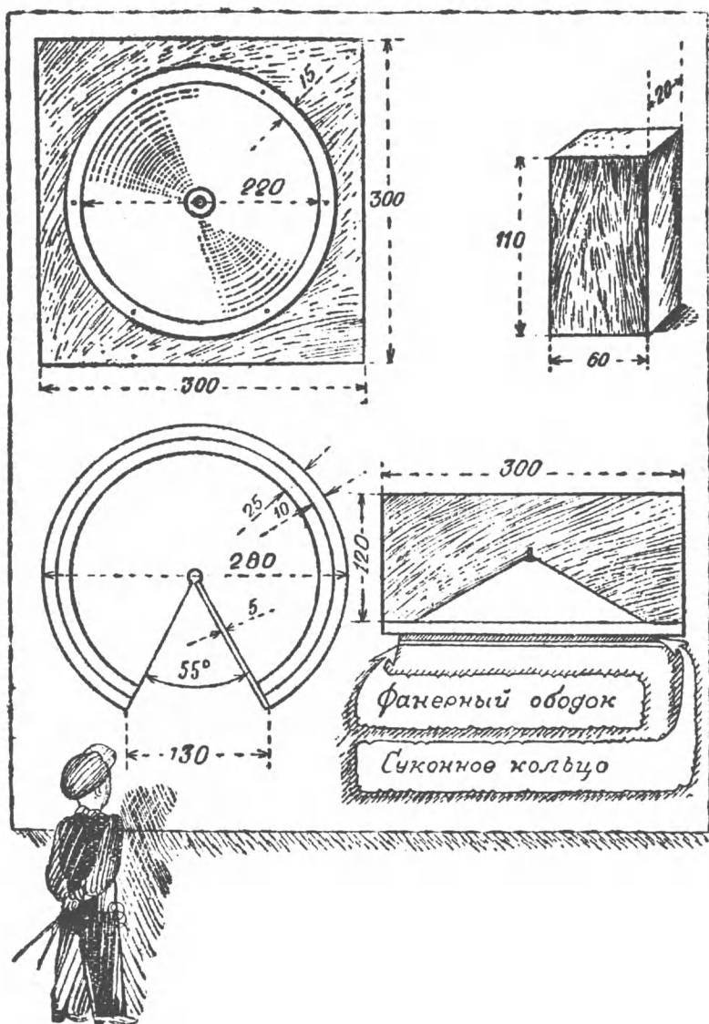
Рис. 48. Конусный диффузор.
