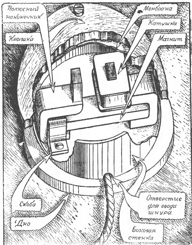
Рис. 36. Общий вид самодельной телефонной трубки.
