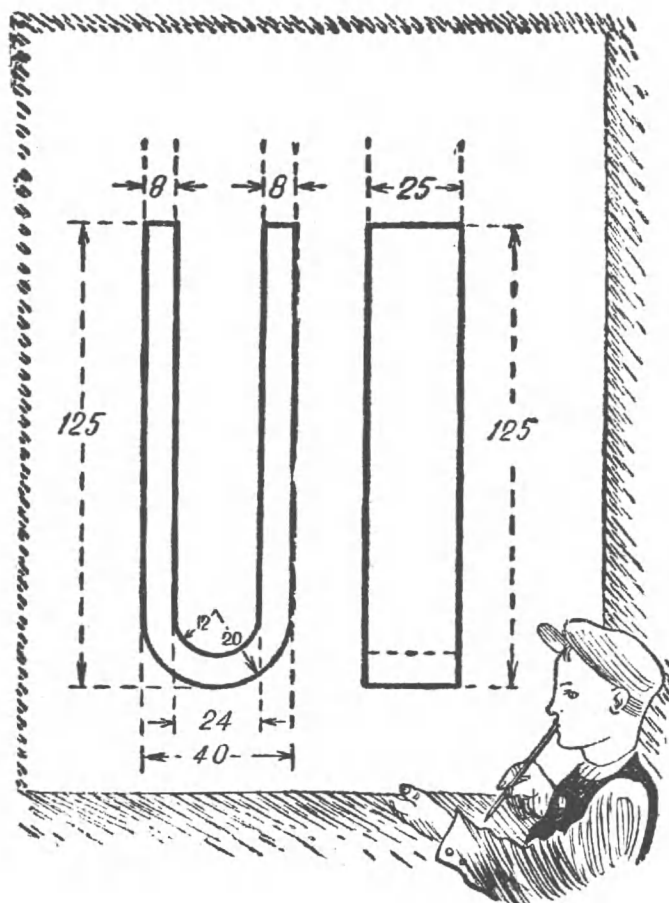
Рис. 54. Магнит для громкоговорителя «Ф-3».
