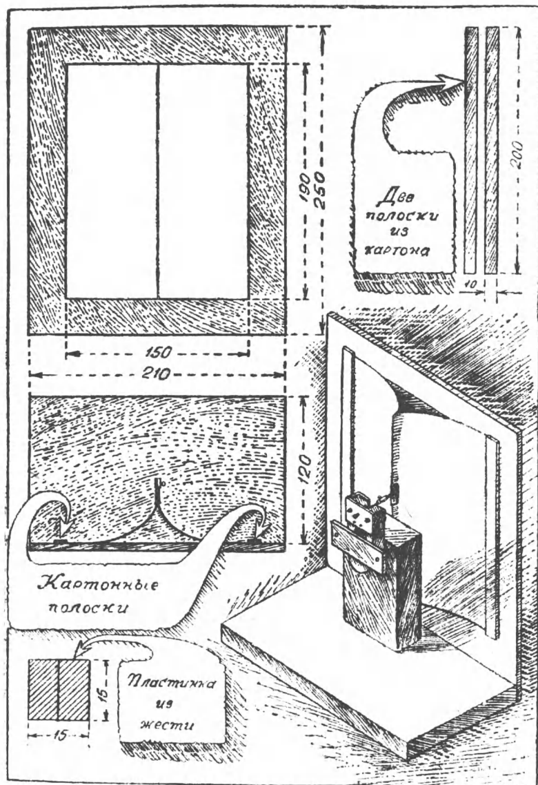
Рис. 47. Диффузор-книжка.
