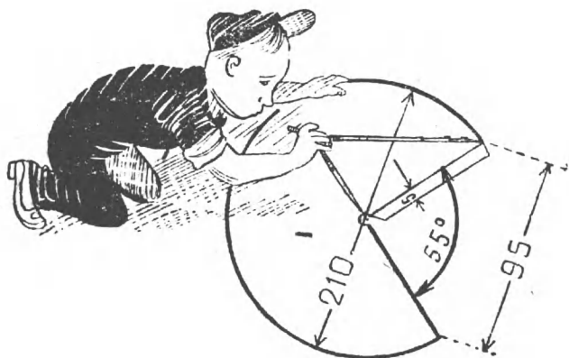
Рис. 23. Выкройка диффузора.
