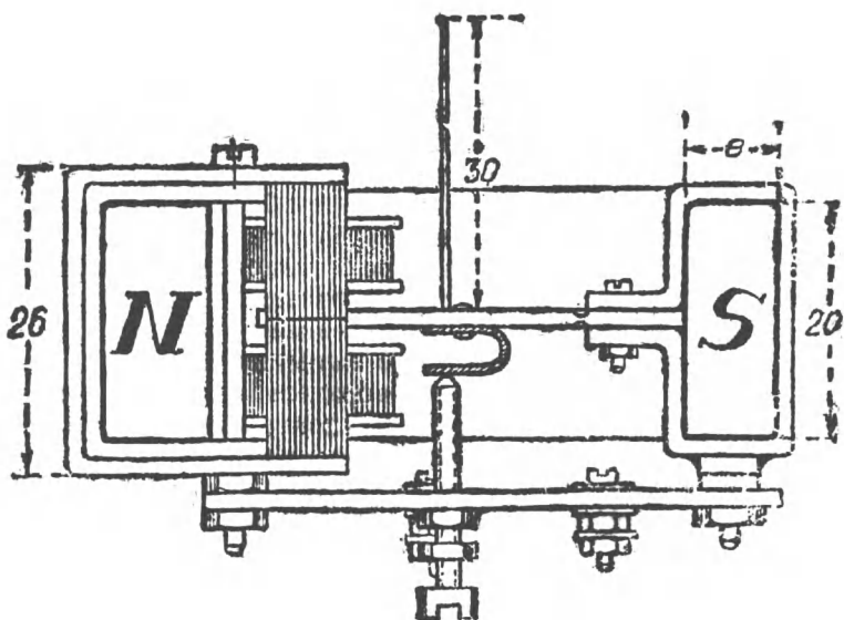
Рис. 43. Вид на механизмы «Рекорд» с торцов магнита.
