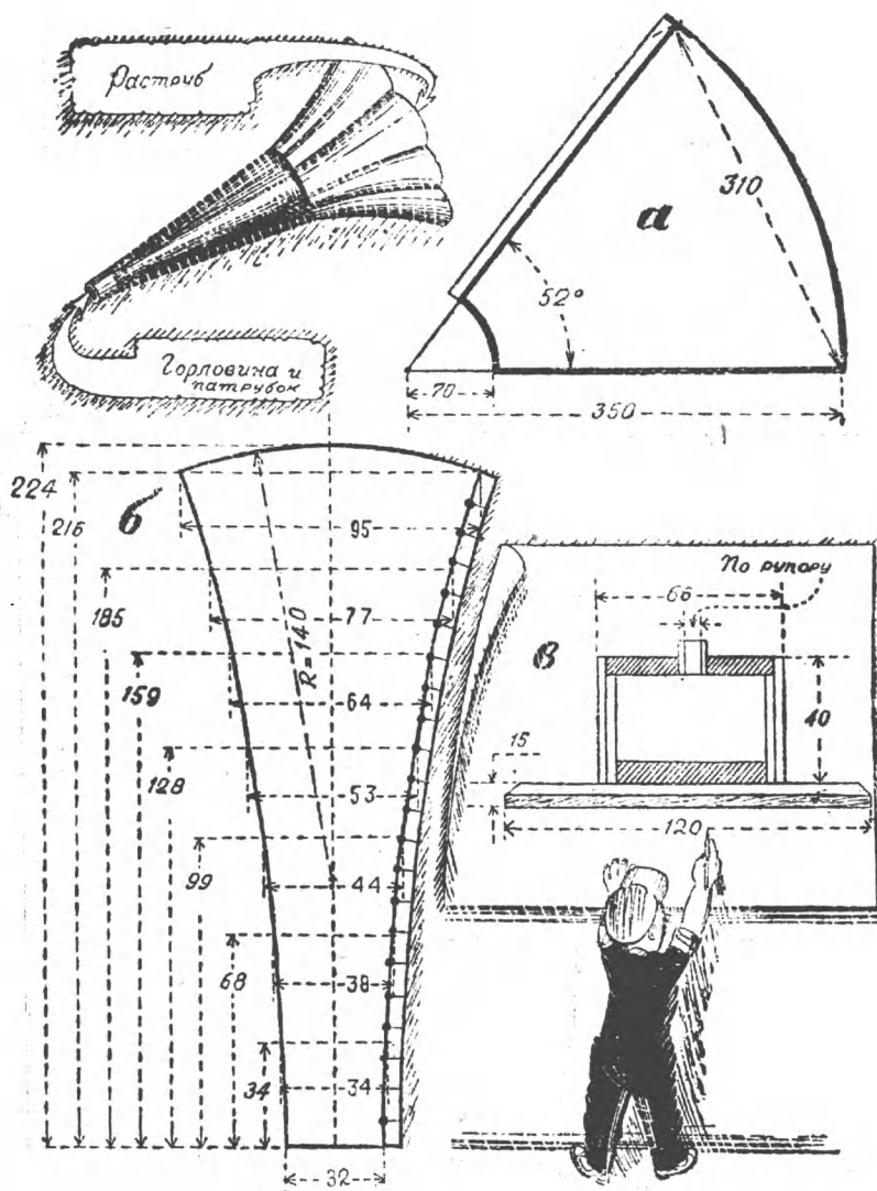
Рис. 19. Прямой рупор и его детали.
