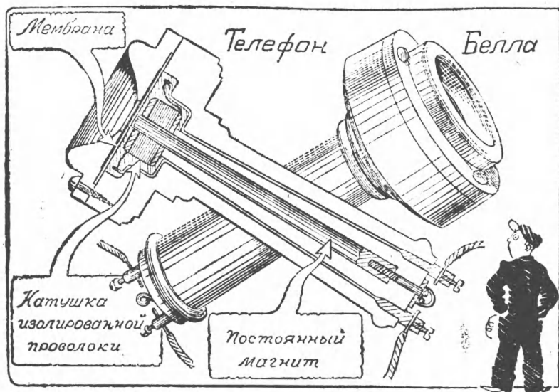
Рис. 10. Телефон Белла.
