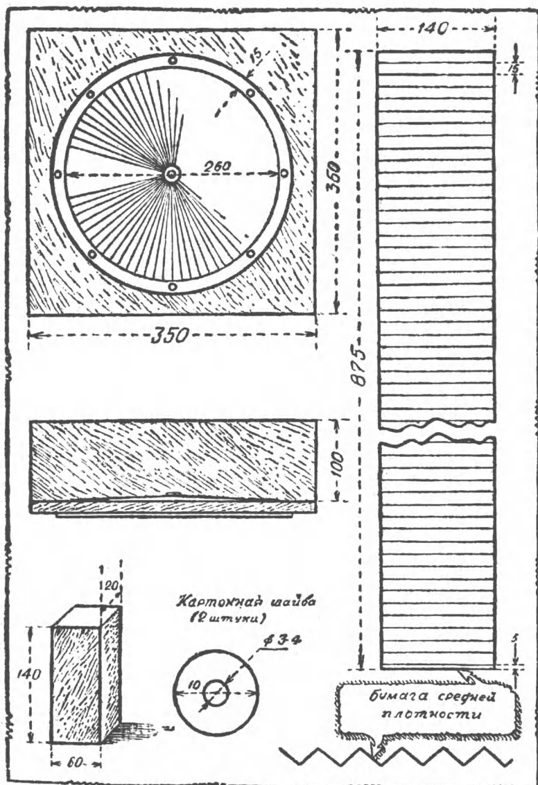
Рис. 49. Веерообразный диффузор.
